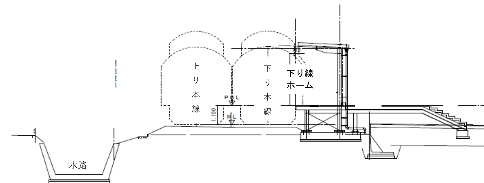
下り線ホーム断面図
