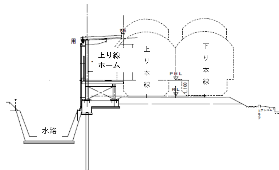
上り線ホーム断面図
