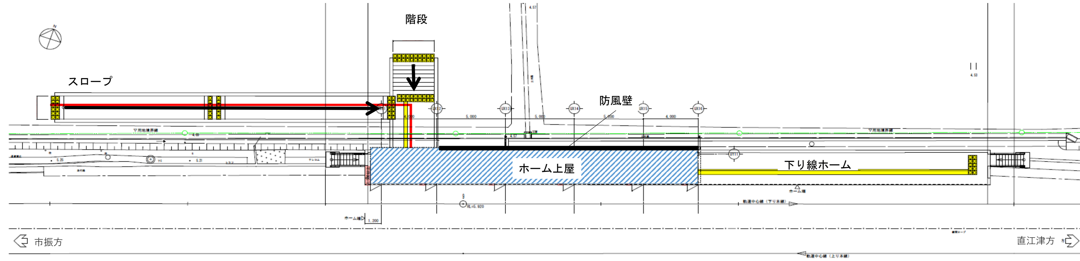
下り線ホーム平面図
