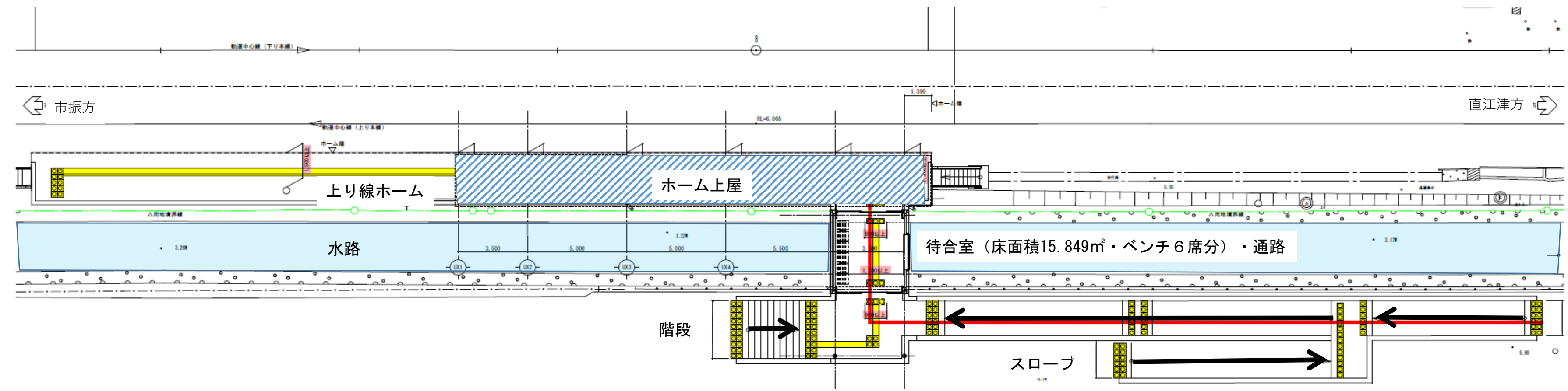
上り線ホーム平面図
